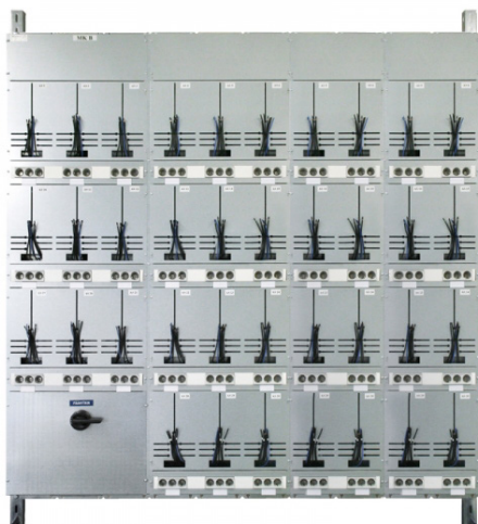
MONIMITTARIKESKUS FFE MMK 34-37 (A/Y) Snro. 3312208 Koko 2000x1970x110mm Väri alumiini https://www.pok.fi/fi/tk/3312208
